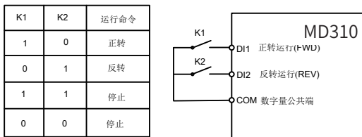
图 6-12 两线式模式 1
