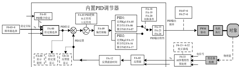
图 4-20 过程控制的频率闭环控制
