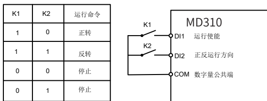
图 6-13 两线式模式 2
