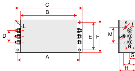
图 7-4 竖力滤波器 DL-25EBK5/ DL-35EBK5/ DL-50EBK5 尺寸图
