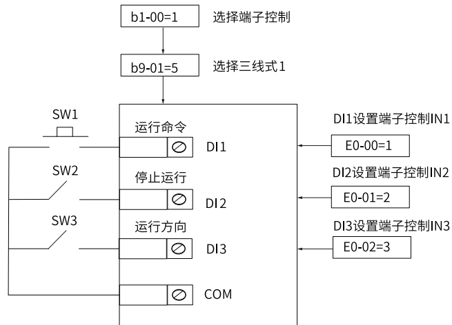
图2-15 三线式模式1接线和参数设置示意图
