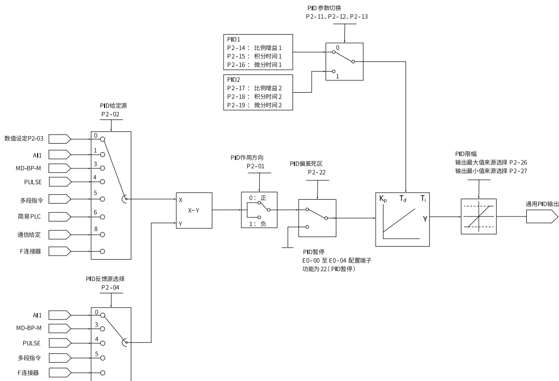
图6-18 通用PID控制参数设置框图
