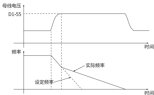
图5-5 过压抑制过程示意图
