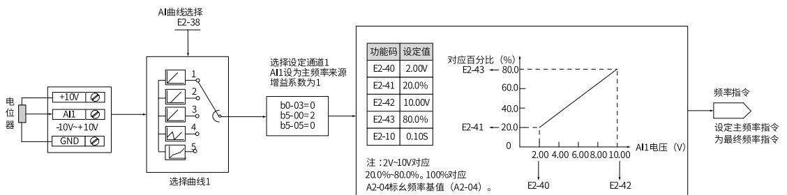
图2-26 AI1电压型输入给定主频率参数设置
