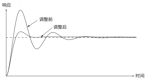
图6-23 增大 T_i 调整趋势图
