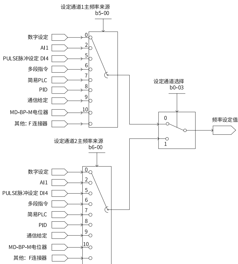
图2-19 设定通道流程图
