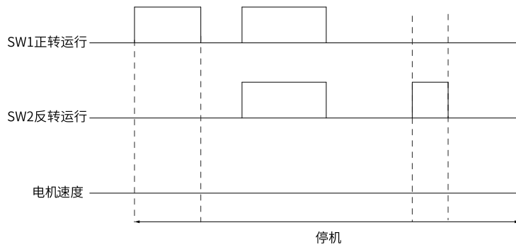
图2-11 两线模式2时序图（异常情况）
