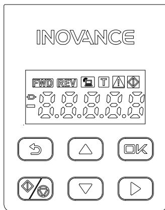
图2-4 6键LED小键盘
