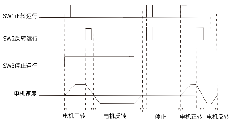
图2-18 三线模式2时序图
