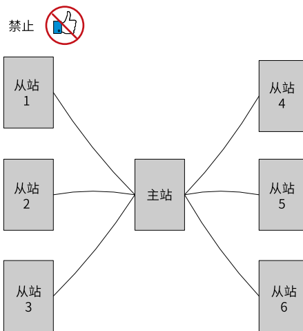
图9-4 星型接线方式（禁止使用）
