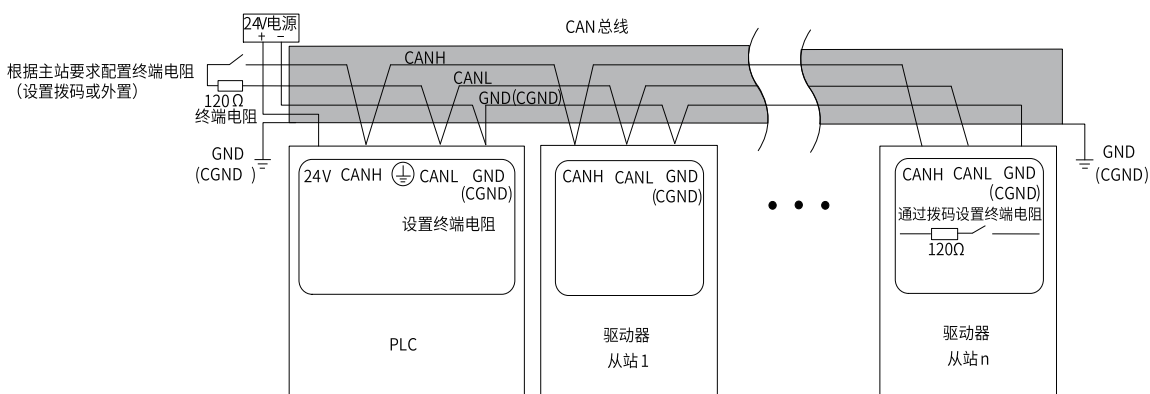
图9-9 CAN总线连接拓扑结构
