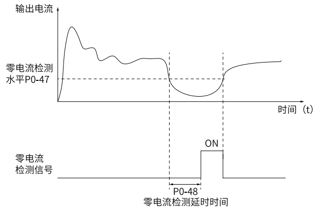
图6-7 零电流检测示意图
