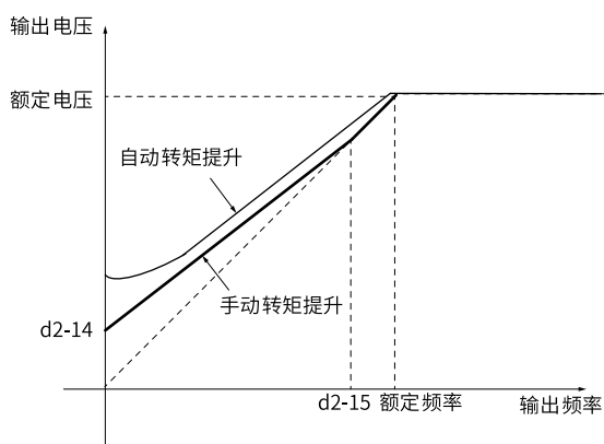
图5-1 直线V/F开启转矩提升时的输出电压和频率示意图
