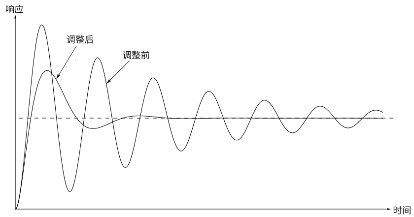
图6-26 加入 T_d 调整趋势图
