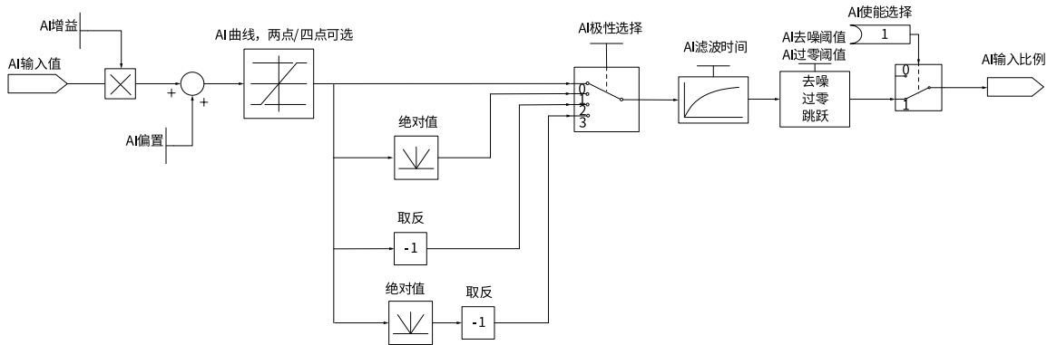
图4-6 模拟输入端子AI逻辑数据流程图
