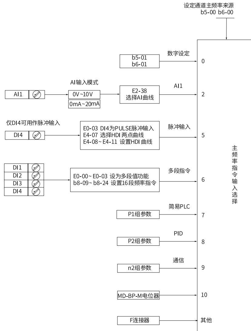
图2-21 主频率指令选择示意图
