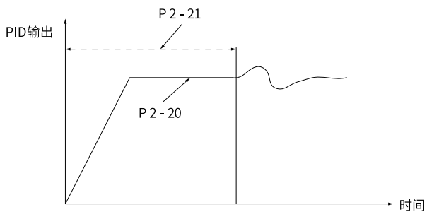
图6-20 PID初值功能示意图
