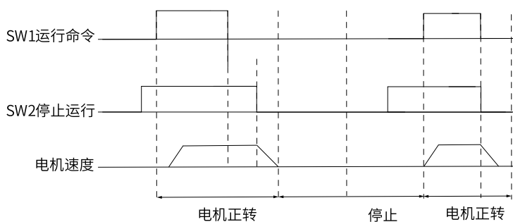
图2-13 两线模式3 时序图（正常情况）
