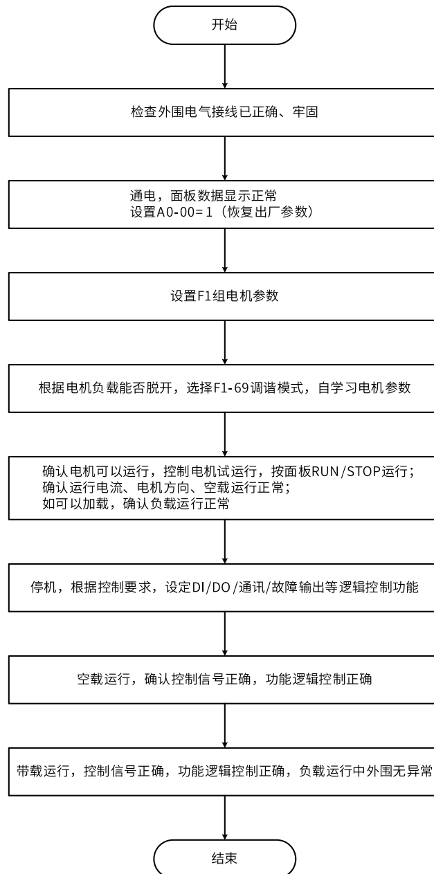
图3-1 快速调试总流程
