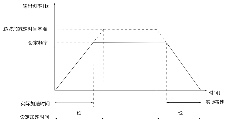
图2-47 加减速时间示意图
