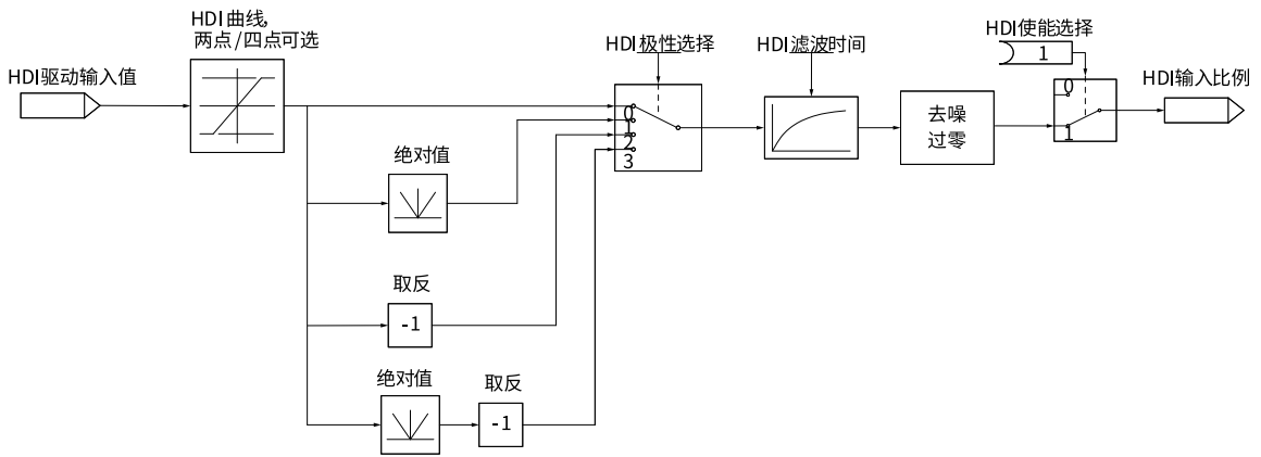
图4-5 高速输入端子HDI数据流程图
