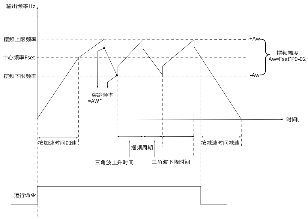
图6-13 摆频工作示意图
