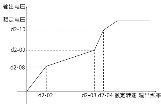
图5-2 多点V/F曲线输出电压和频率示意图
