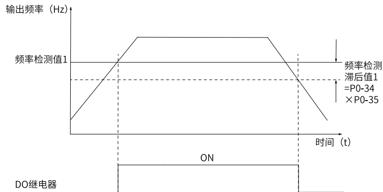
图6-2 频率检测示意图
