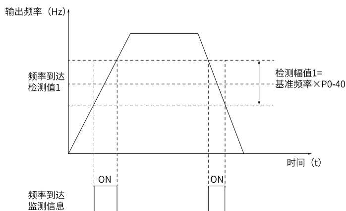
图6-6 任意到达频率检测示意图
