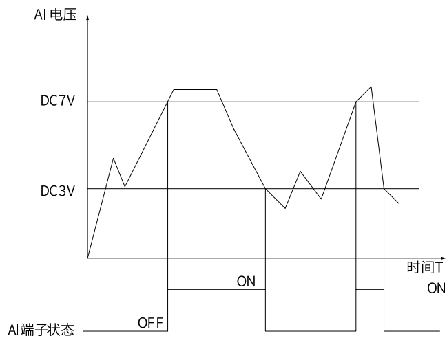
图4-7 AI输入电压与DI状态的关系图
