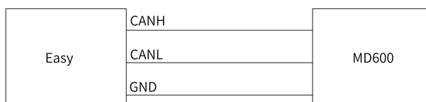
图9-7 通信口连接
