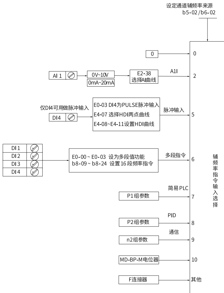
图2-36 辅助频率给定来源选择示意图
