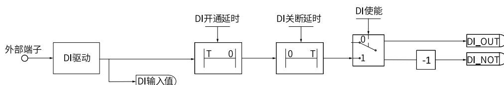
图4-1 输入端子DI逻辑数据流程图
