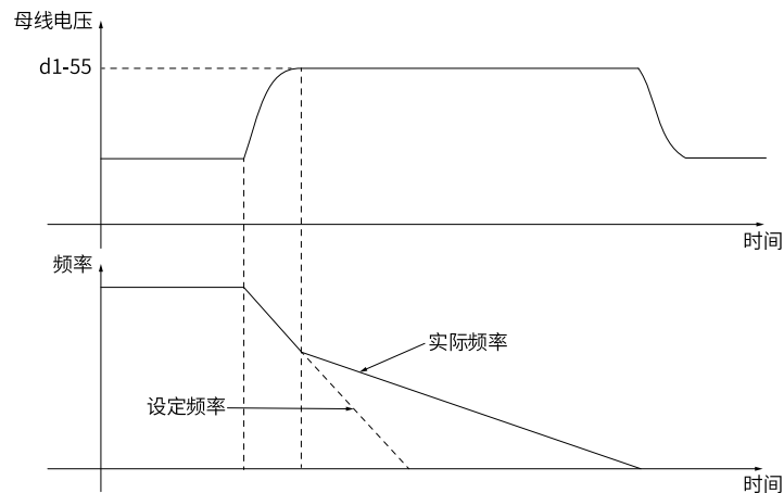
图7-1 过压抑制过程示意图
