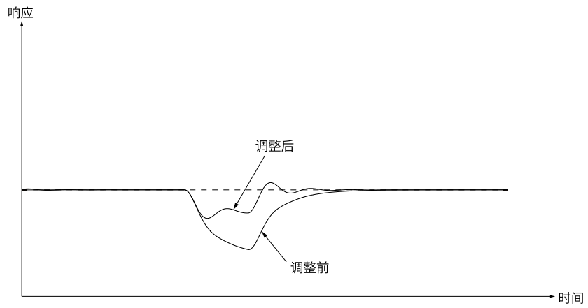
图6-25 负载波动时，减小Ti调整趋势图
