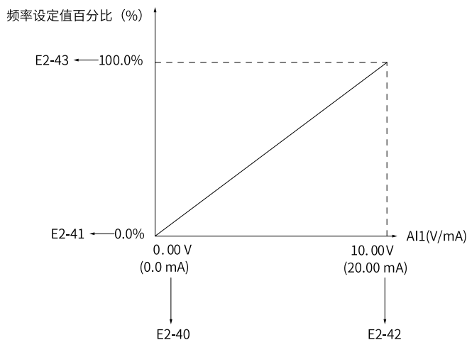
图2-23 曲线1设定示意图
