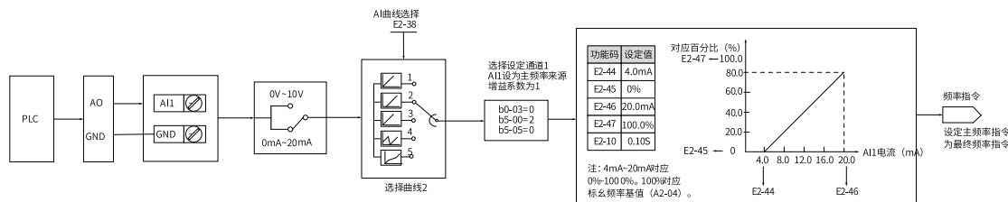
图2-27 AI1电流输入给定主频率参数设置
