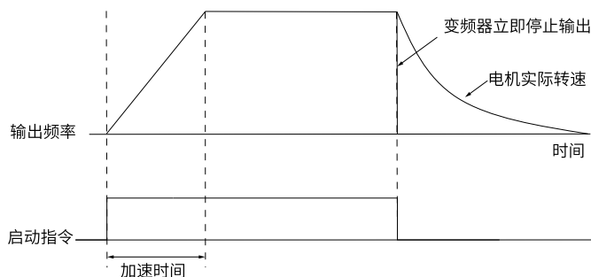
图2-45 自由停车时序图
