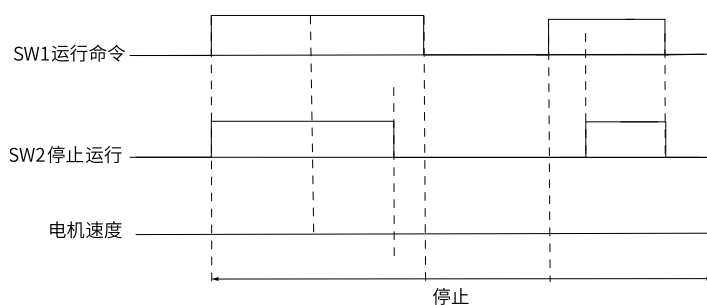
图2-14 两线模式3时序图（异常情况）
