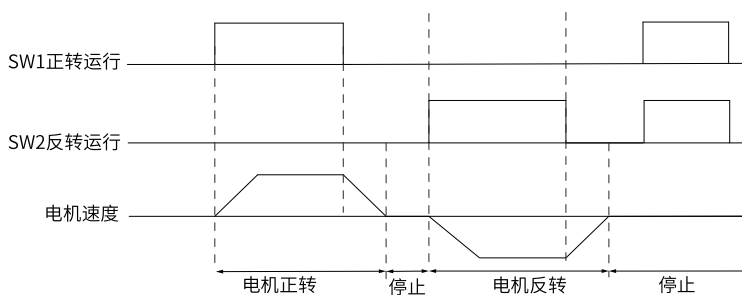
图2-10 两线模式2 时序图（正常情况）
