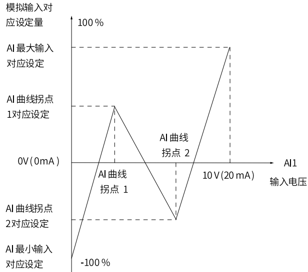
图2-25 曲线4和曲线5示意图
