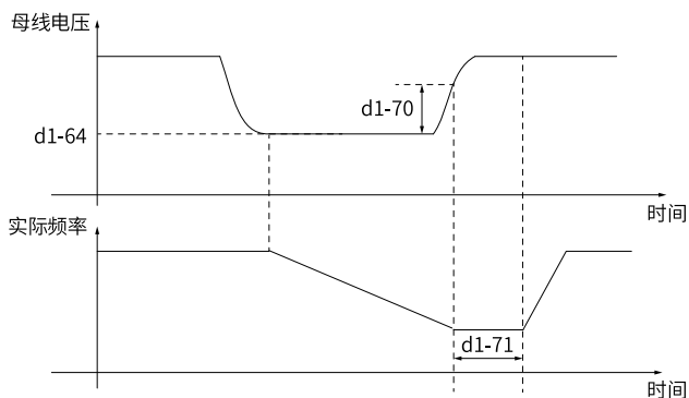
图7-2 欠压抑制模式示意图
