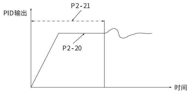
图2-33 PID初值功能示意图
