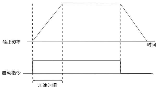
图2-39 直接启动时序图
