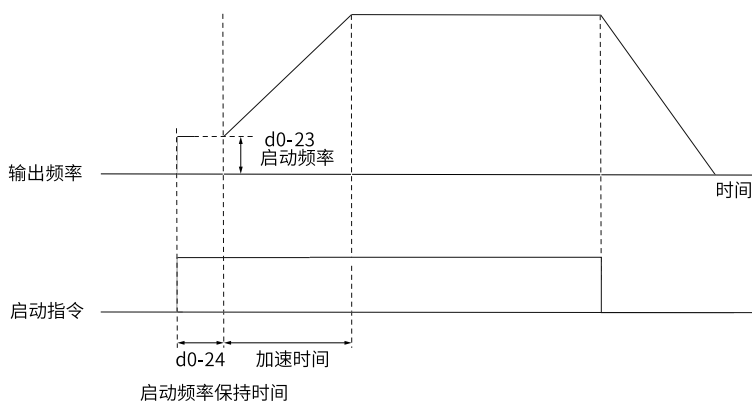
图2-40 带启动频率的启动时序图
