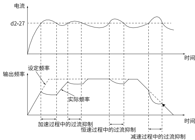
图5-4 电机在加速、恒速、减速过程中的输出电流和频率变化示意图
