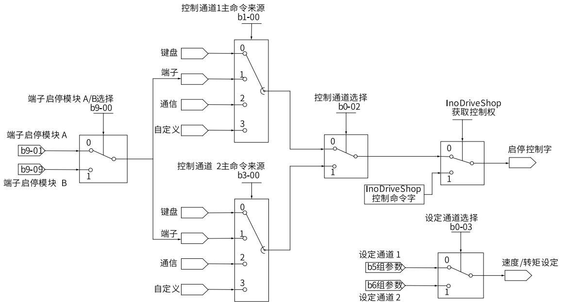
图2-1 指令通道的选择
