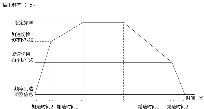
图6-5 加减速时间切换示意图
