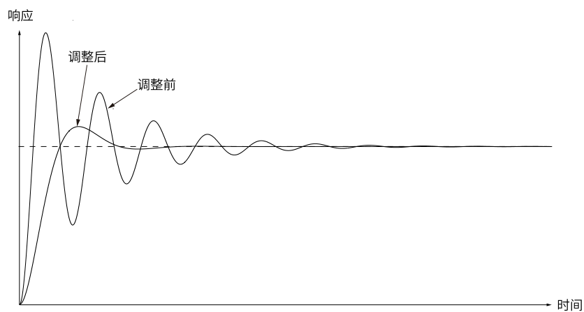
图6-22 减小 K_p 调整趋势图
