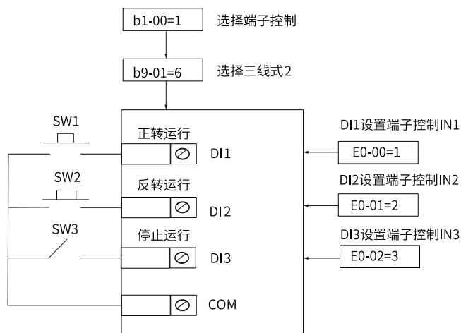
图2-17 三线式模式2接线和参数设置示意图
