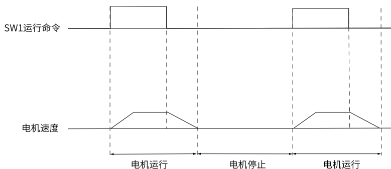
图2-6 一线模式时序图
