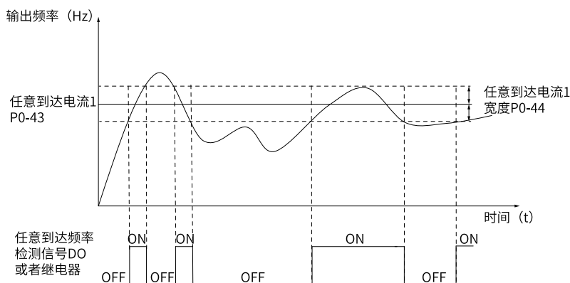
图6-9 任意到达电流时序图
