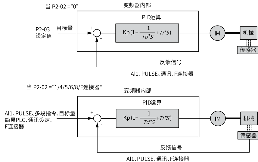
图2-30 过程PID控制原理框图
