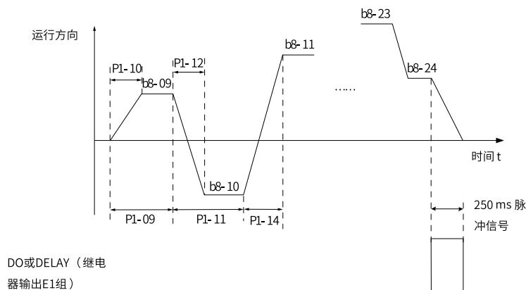
图2-29 简易PLC作为主频率示意图
