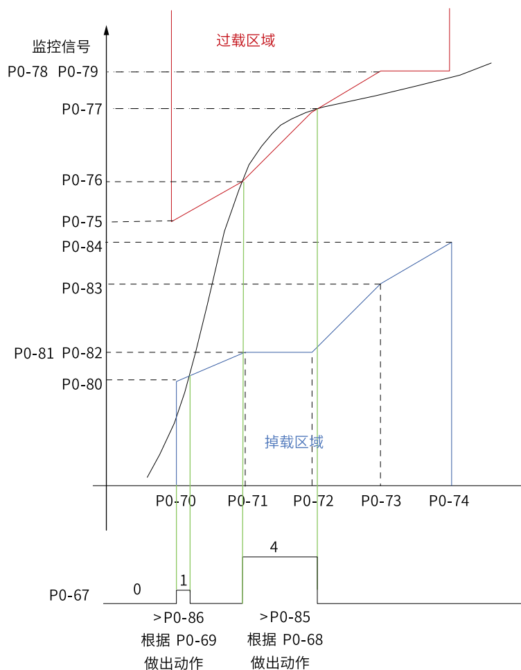
图6-27 负载监控及响应动作原理示意图
