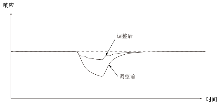
图6-24 负载波动时，增大Kp调整趋势图
