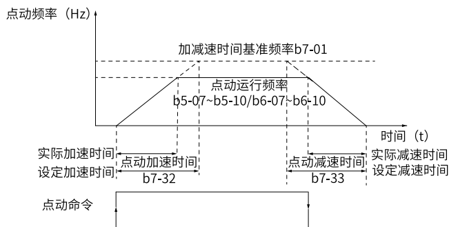
图6-1 点动运行示意图
