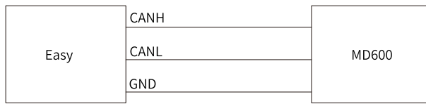
图9-10 通信口连接
