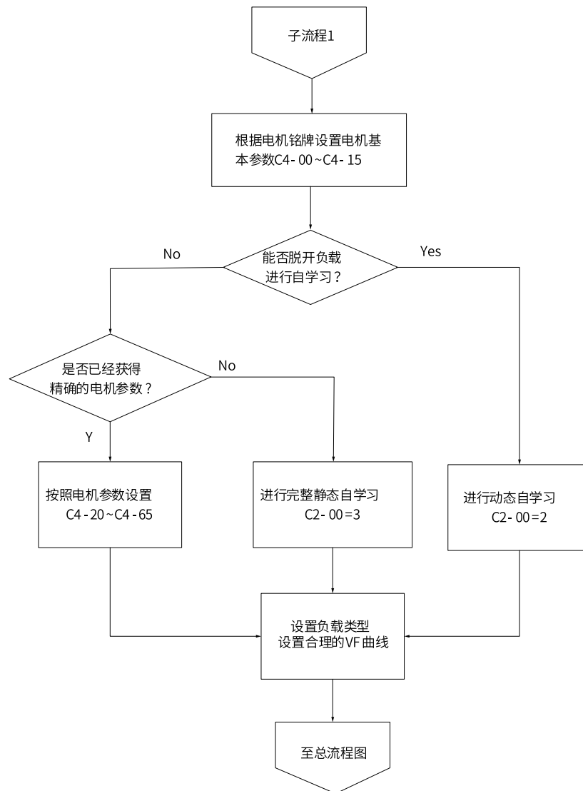
图3-3 变频器调试子流程图1 (V/F控制)
