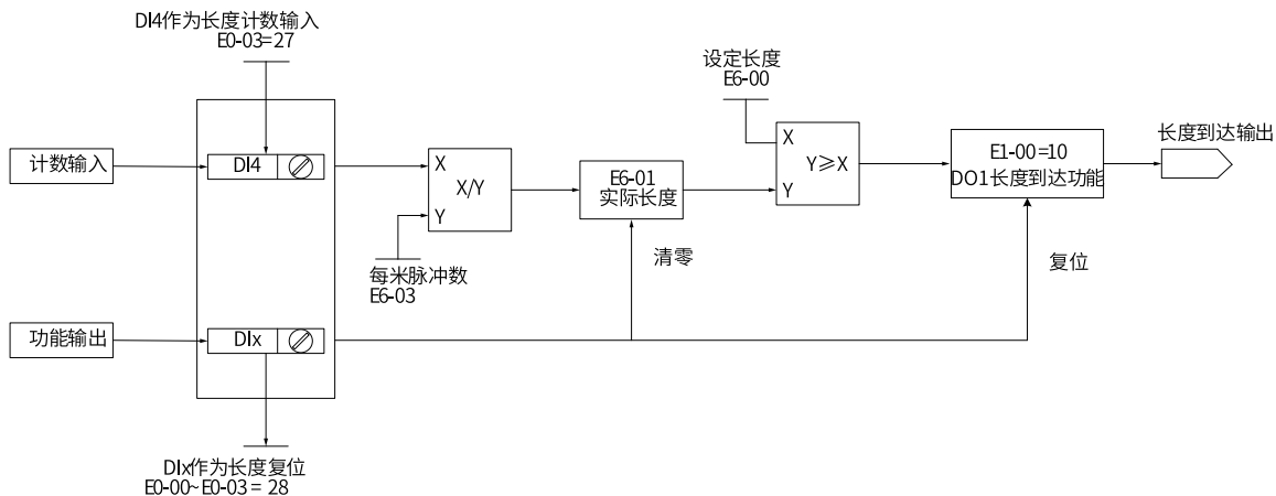
图6-14 定长功能示意图
