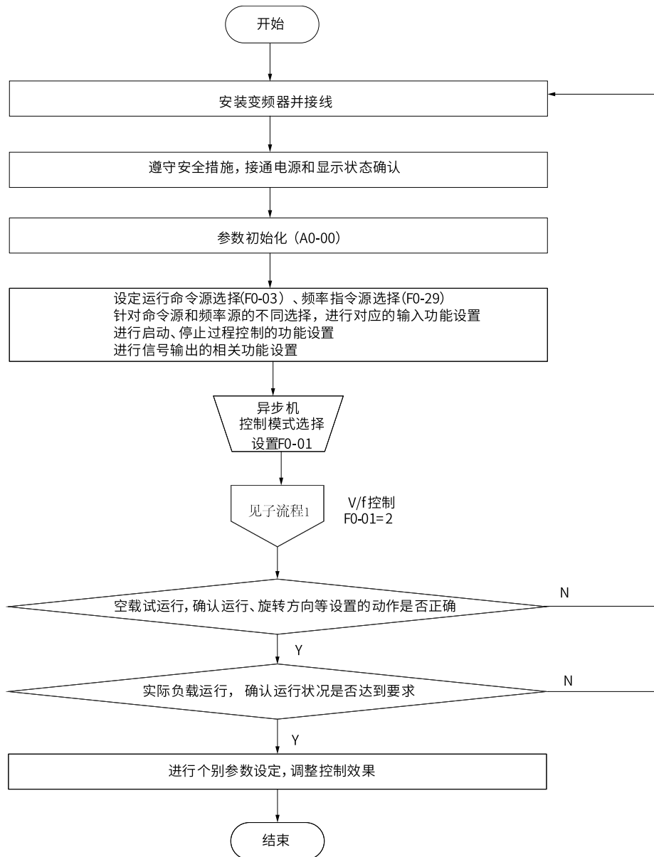
图3-2 调试总流程图
