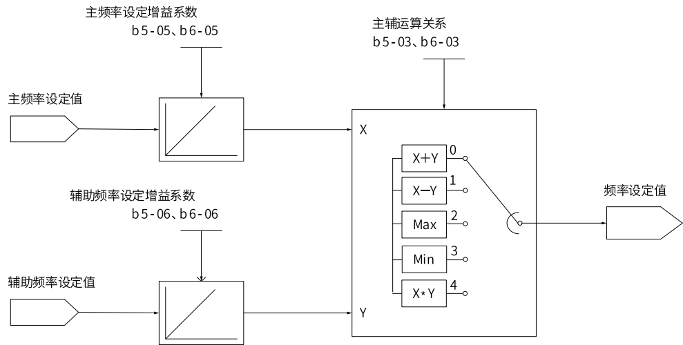
图2-20 主辅频率指令输入示意图
