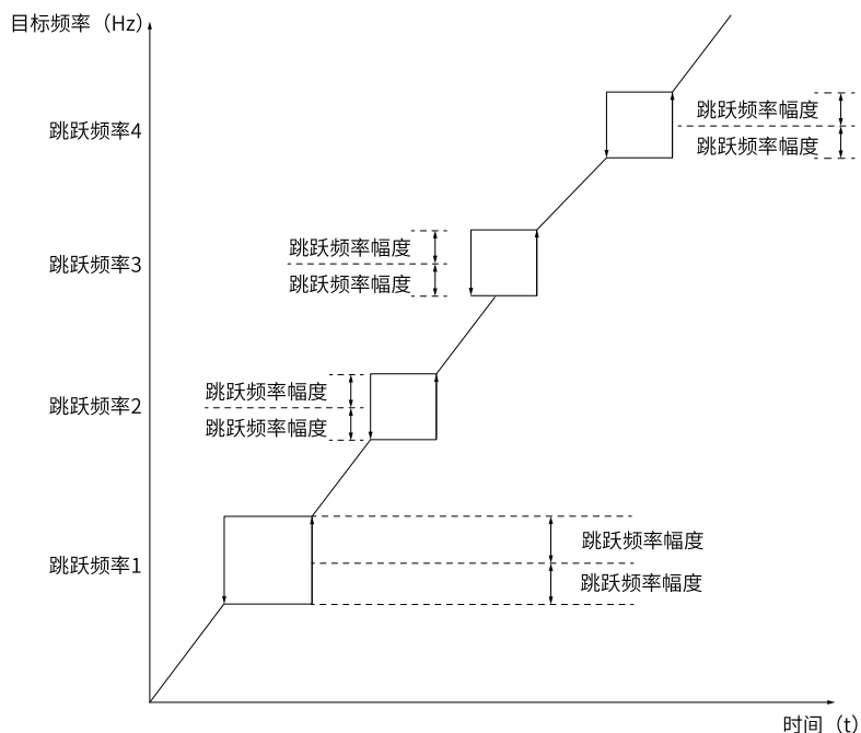
图6-3 跳跃频率示意图
