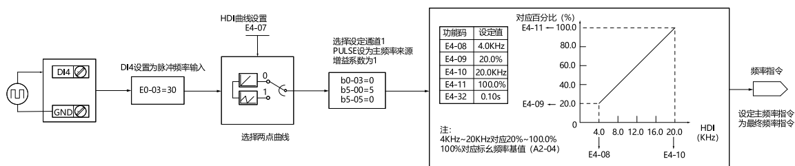
图2-35 脉冲输入给定主频率参数设置
