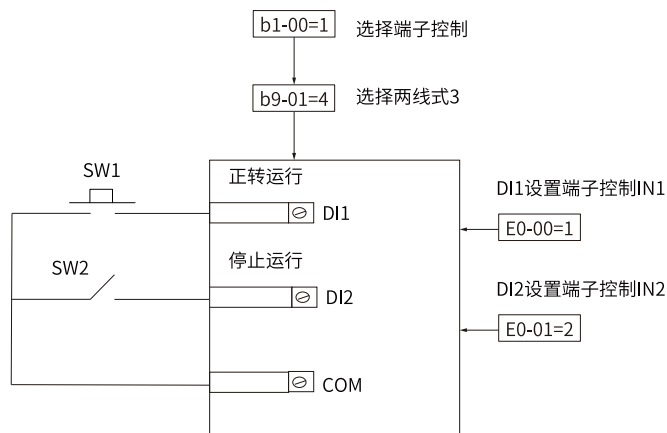
图2-12 两线式模式3接线和参数设置示意图
