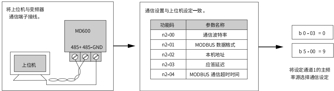
图2-34 通信设定作为主频率设置
