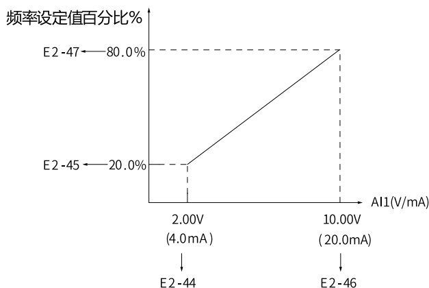
图2-24 曲线2设定示意图
