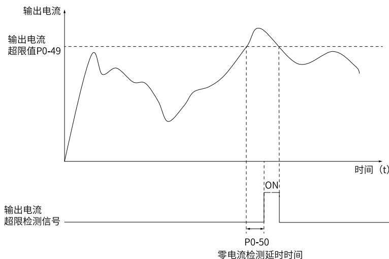
图6-8 输出电流超限检测示意图
