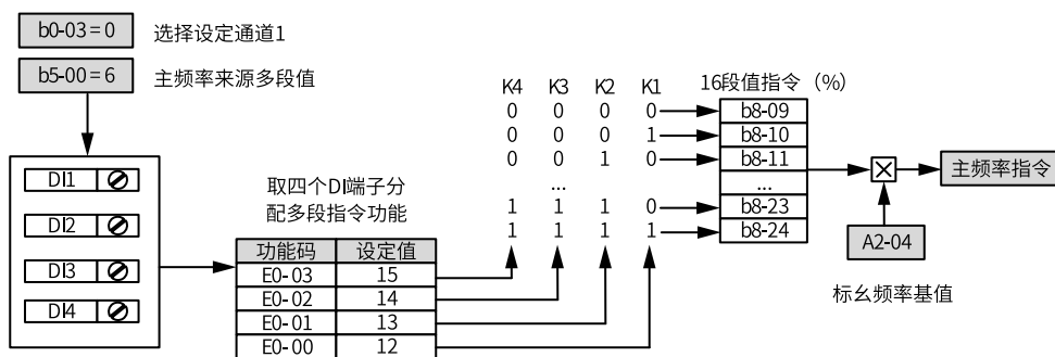
图2-28 多段速模式的设置
