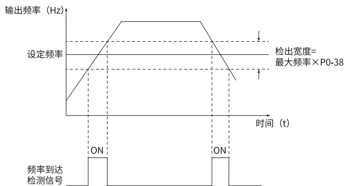
图6-4 频率到达检出幅值时序图
