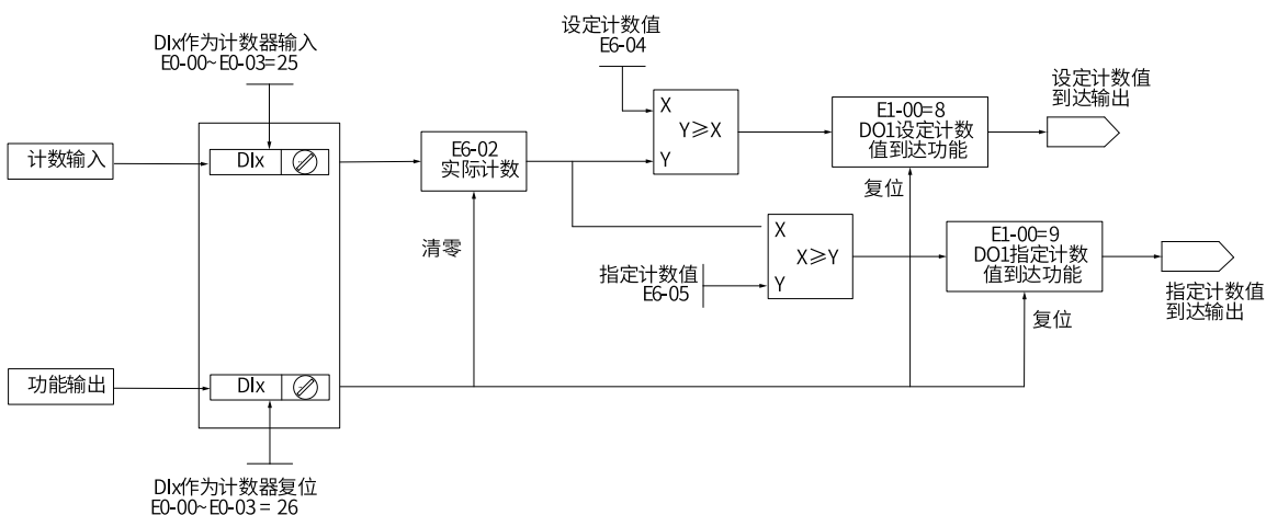
图6-15 计数功能示意图
