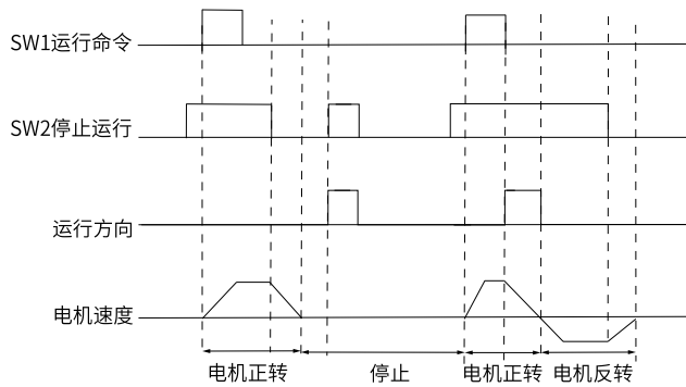
图2-16 三线模式1 时序图
