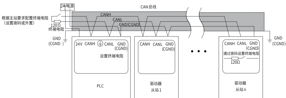
图9-6 CAN总线连接拓扑结构
