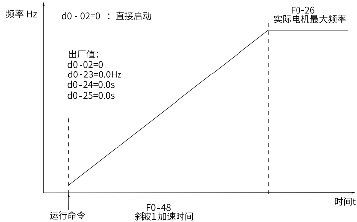
图2-42 直接启动方式
