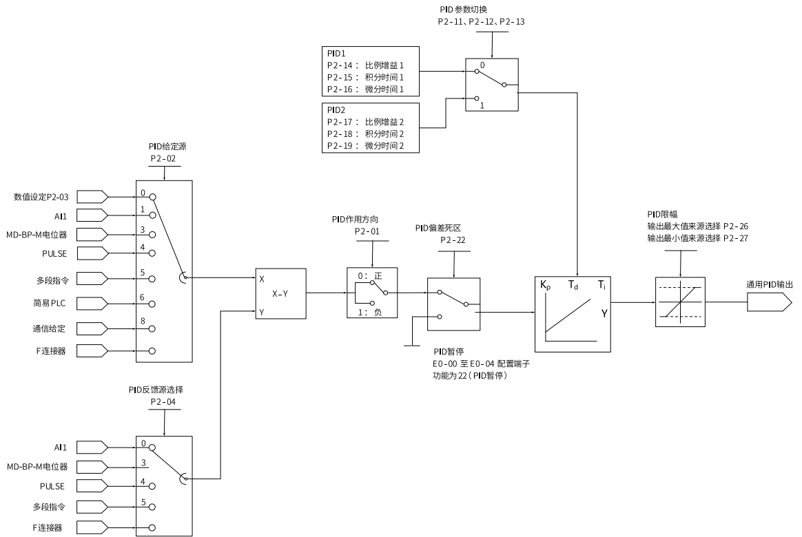
图2-31 过程PID控制参数设置框图
