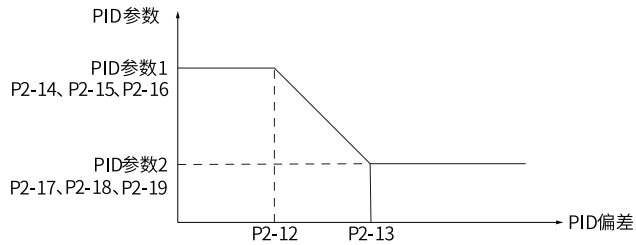
图2-32 PID参数切换
