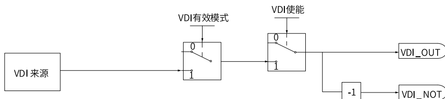
图4-3 虚拟输入端子VDI数据流程图
