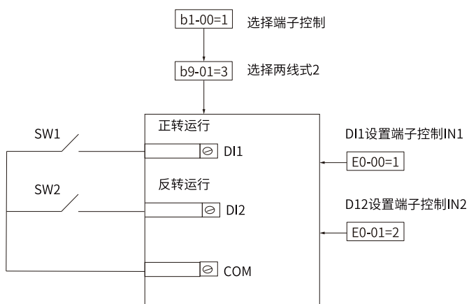
图2-9 两线式模式2接线和参数设置示意图
