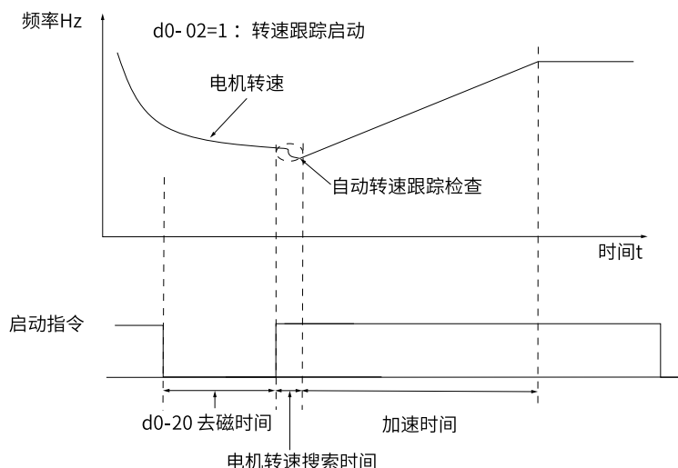
图2-43 转速跟踪启动
