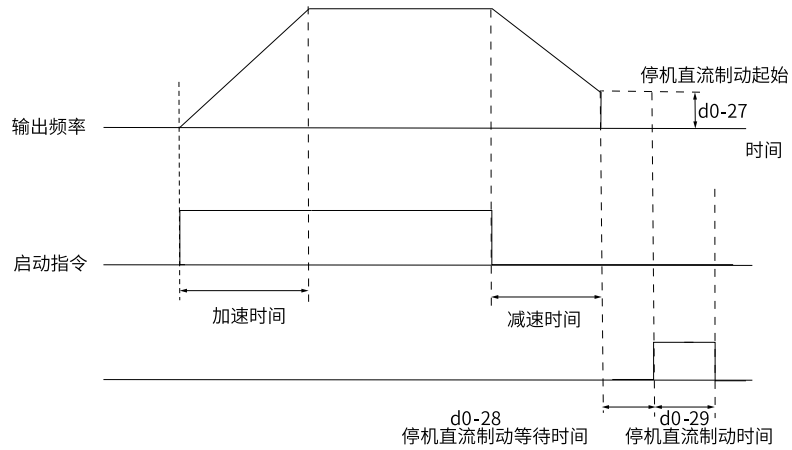
图2-46 停车直流制动时序图
