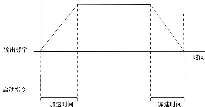
图2-44 减速停车时序图
