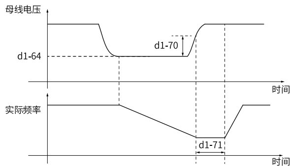
图5-6 欠压抑制模式示意图
