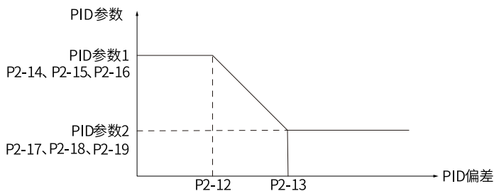
图6-19 PID参数切换
