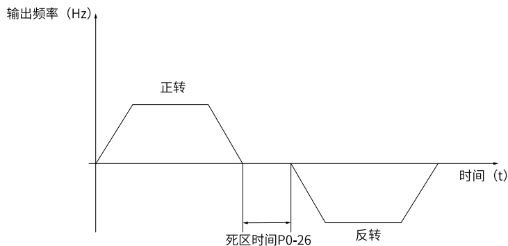
图6-10 正反转死区时间示意图
