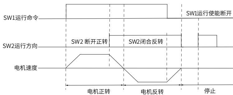
图2-8 两线模式1时序图
