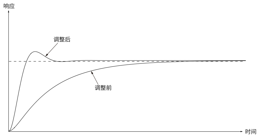
图6-21 增大 K_p 调整趋势图
