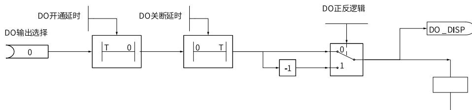
图4-2 输出端子DO数据流程图
