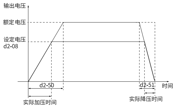
图5-3 V/F分离模式下，电压加减速时间示意图
