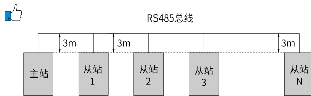
图9-3 采用分支线连接
