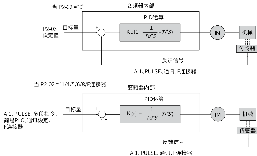
图6-17 通用PID控制原理框图
