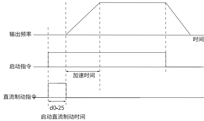
图2-41 带直流制动的启动时序图
