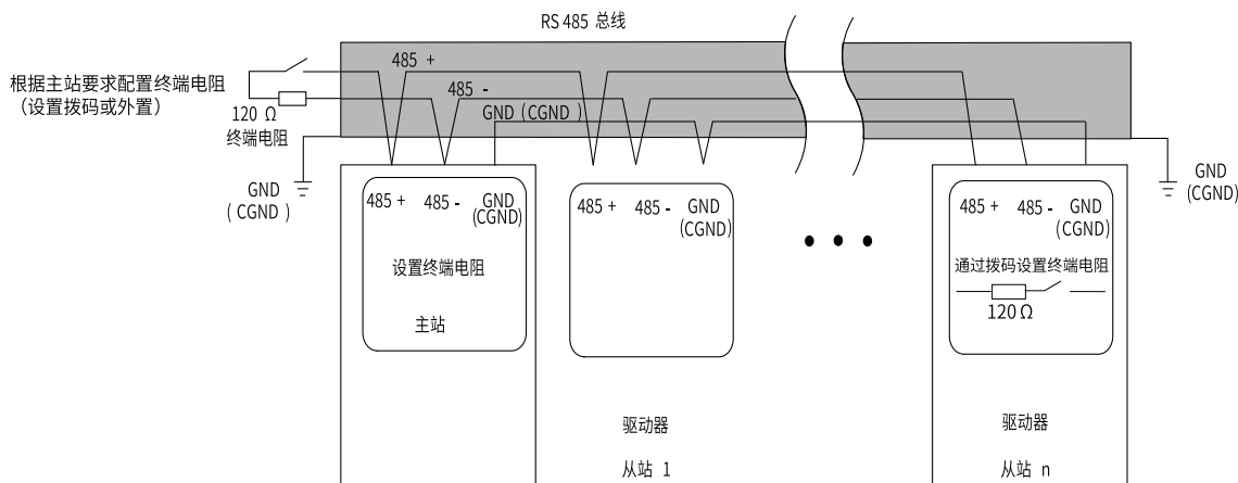
图9-1 RS485总线连接拓扑结构
