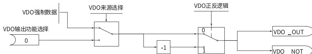
图4-4 虚拟输出端子VDO数据流程图
